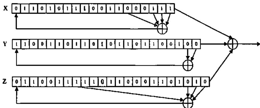
Рис.3.5. Начальное состояние регистров X , Y и Z
