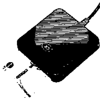
Рис.4.1. Смарт-карта и устройство считывания смарт-карт (ACR39U)
