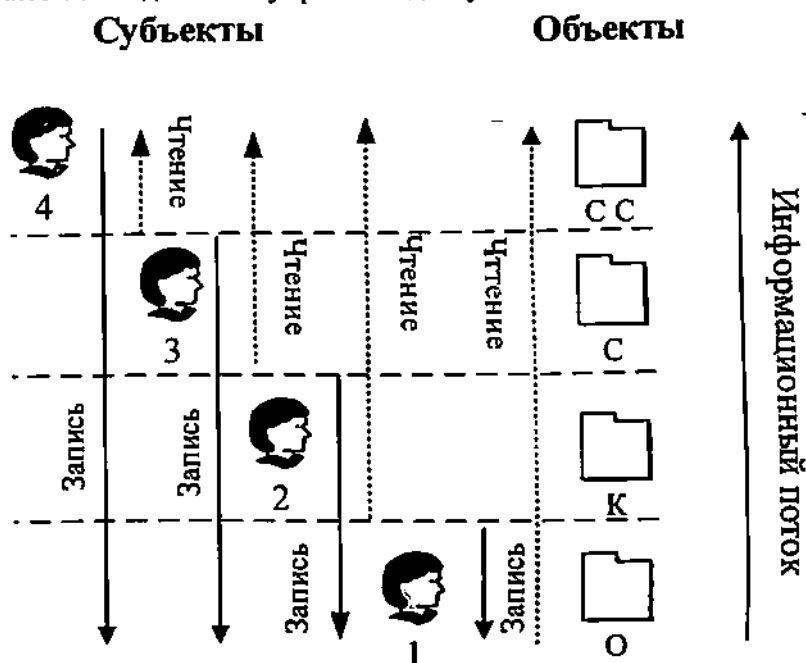
Рис.4.6. Схема управления информационными потоками для обеспечения надежности данных
