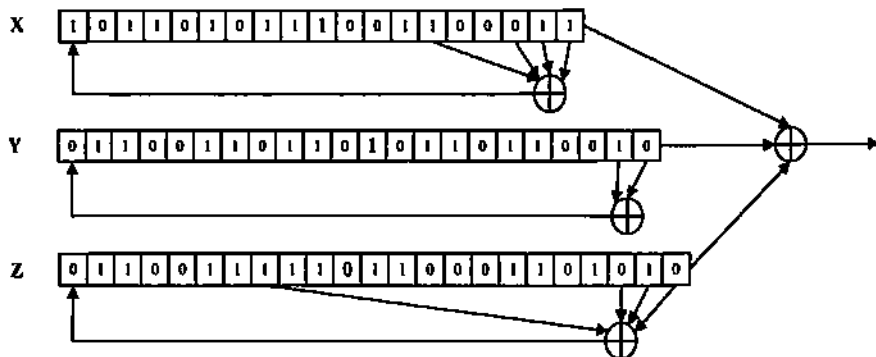
Рис.3.6. Состояние, после сдвига регистров X , Y и Z
