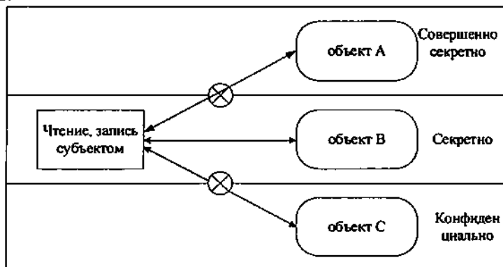
Рис.4.12. Схема информационных потоков для свойства «- Strong Property»
