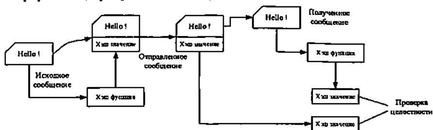
Рис. 3.8. Проверка целостности данных на основе хэш-функции
