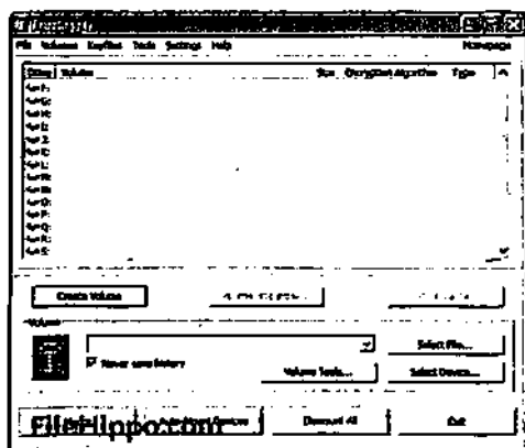
Рис.3.12. Программное средство TrueCrypt
