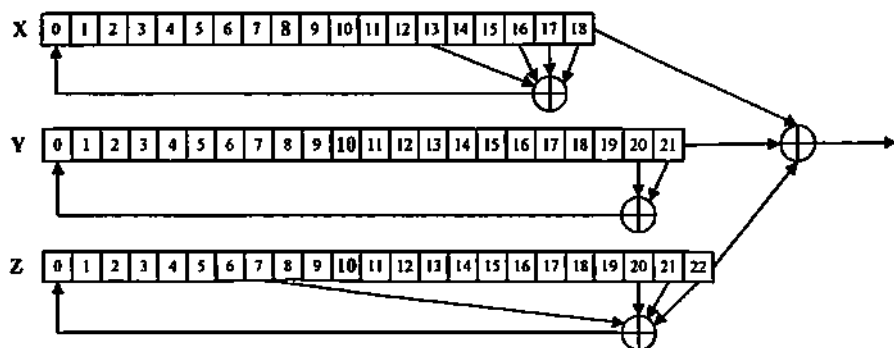
Рис.3.4. Общий вид генератора последовательности А5/1
