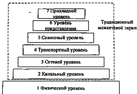
Рис.4.16. Использование межсетевых экранов на сетевых уровнях
