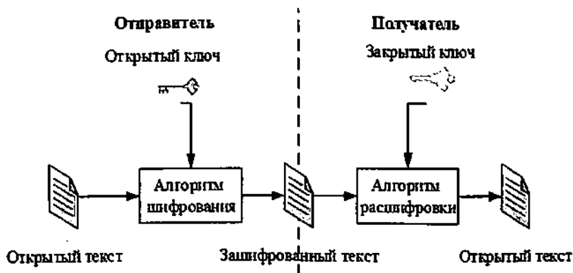
Рис.3.2. Общий вид шифрования с открытым ключом
