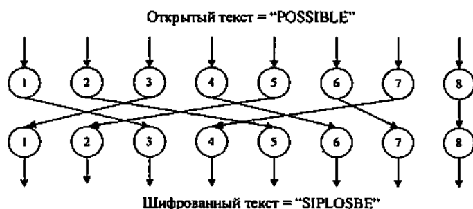
Рис.3.3. Пример простого метода перестановки
